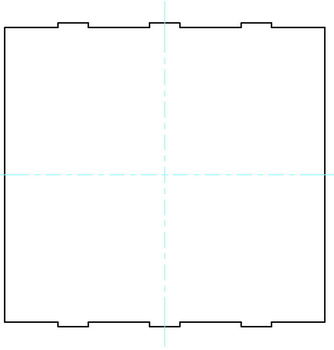
Dパネル2裏面 / D Panel 2 Backside
