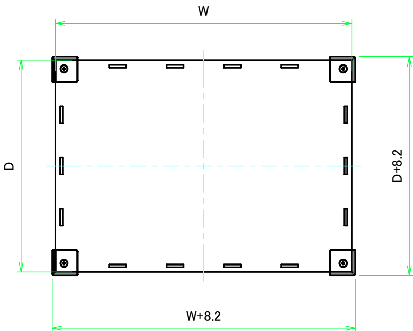
上カバー / Top cover
